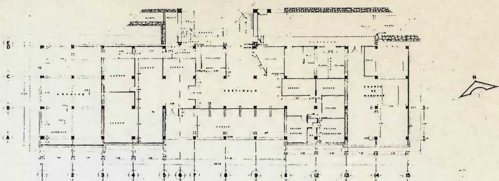
PLANTA ARQUITECTONICA SOTANO
