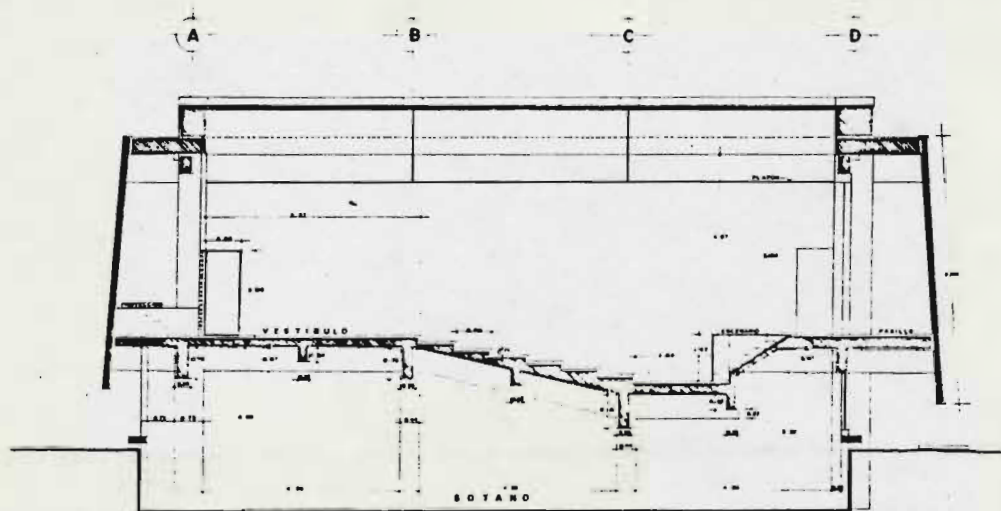
AUDITORIO CORTE B-B' ESC. 1:50
