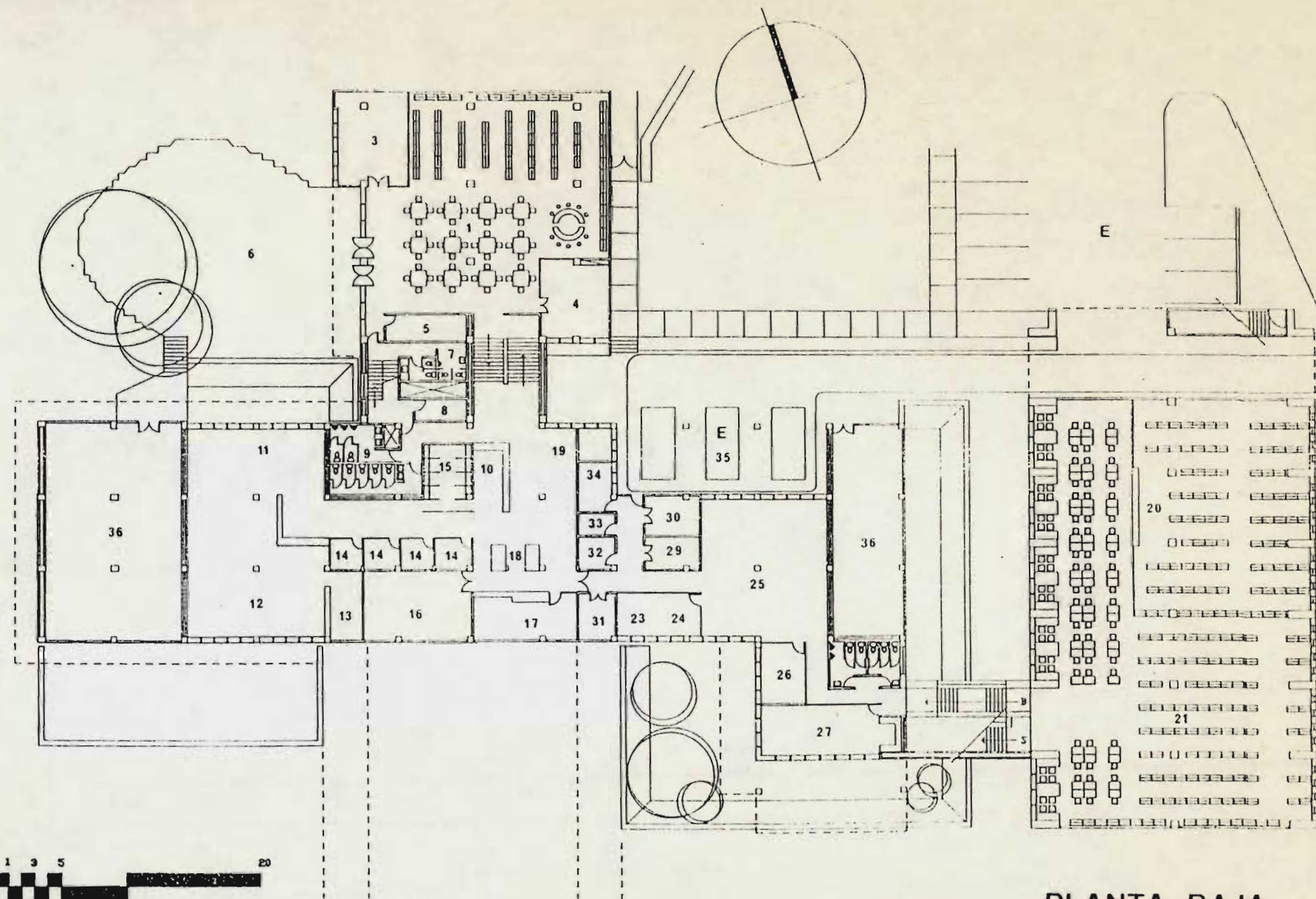
PLANTA BAJA
